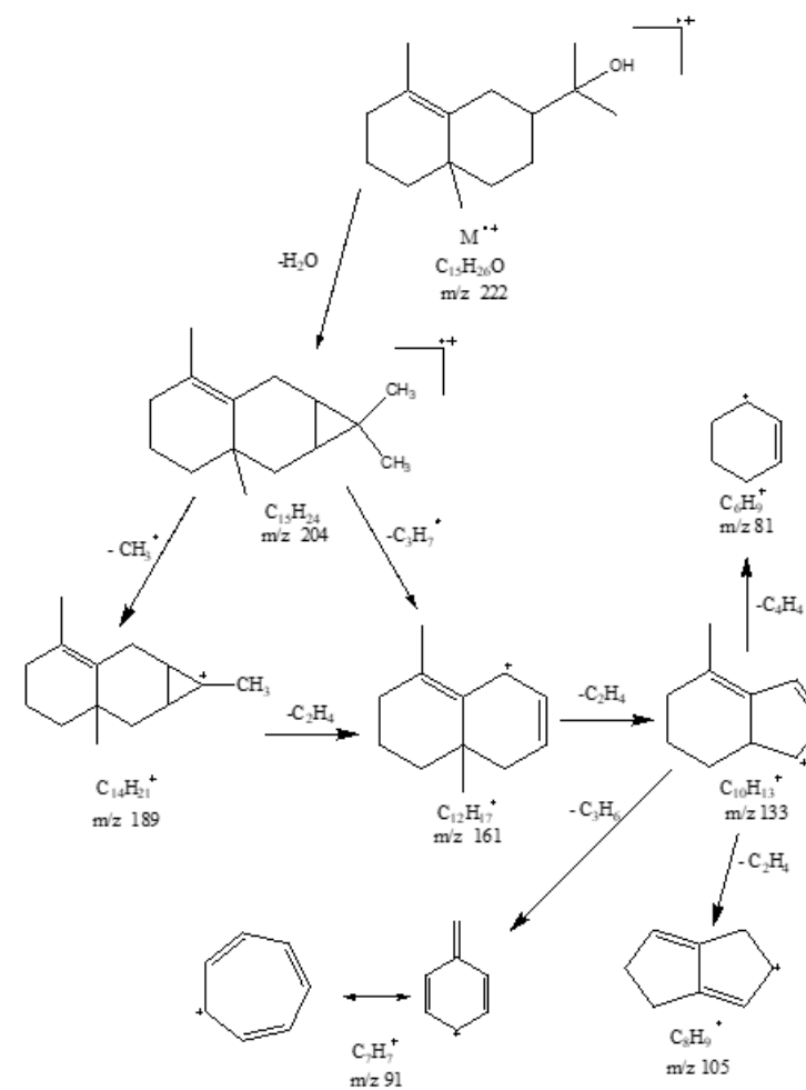
(d) Eudesmol
