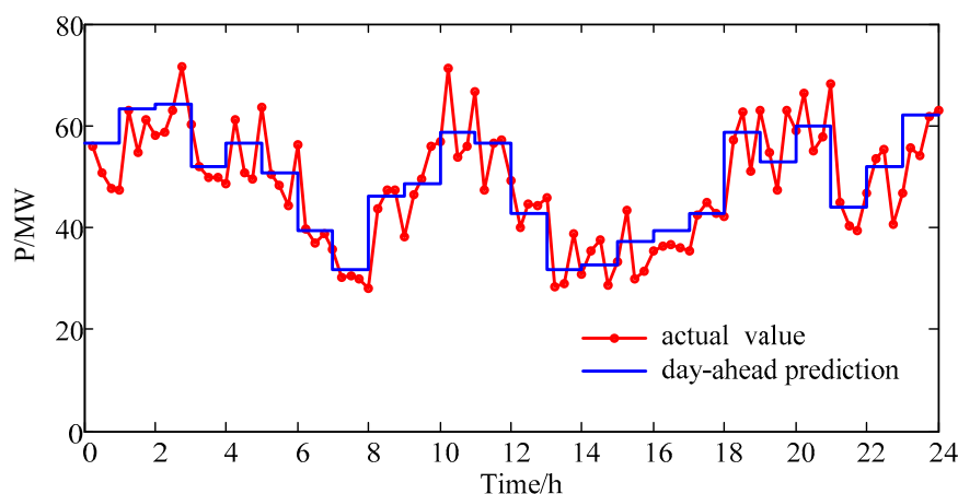
Figure 7. Actual wind power.
